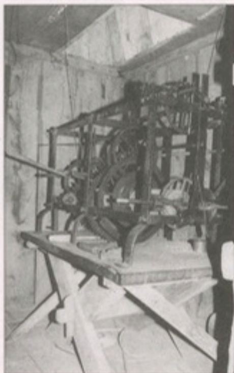
Abb. 1 Die Werke der Uhr des Klosters Marienfeld sind hintereinander angeordnet und mit einem kurzen Pendel versehen. Die Uhr stammt aus dem 17. Jahrhundert, überstand den Brand der Kirche im Jahr 1825 und läuft heute noch (Foto: A. Sassen)
