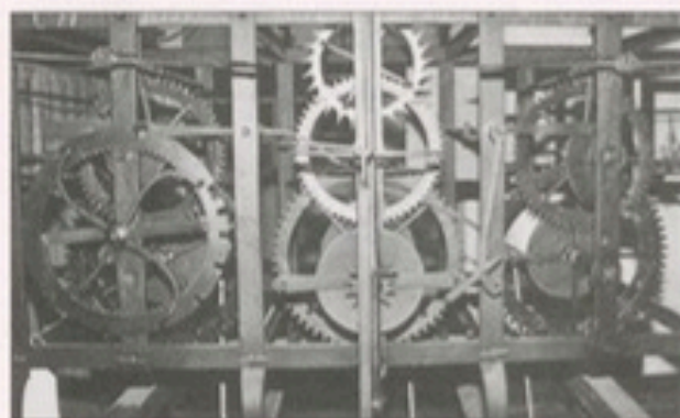
Abb. 2 Die Turmuhr der ev. Kirche zu Isselhorst, heute im Museum des Brennerhofes Elmendorf funktionstüchtig aufgebaut. In der Mitte das Gehwerk der Uhr, rechts das Schlagwerk für die Viertelstunden, links das Schlagwerk für die Vollstunden. Am oberen Riegel des verkeilten Eisenrahmens ist die Signatur des Uhrbauers Rieke aus Halle von 1735 zu sehen (Foto: A. Sassen)
