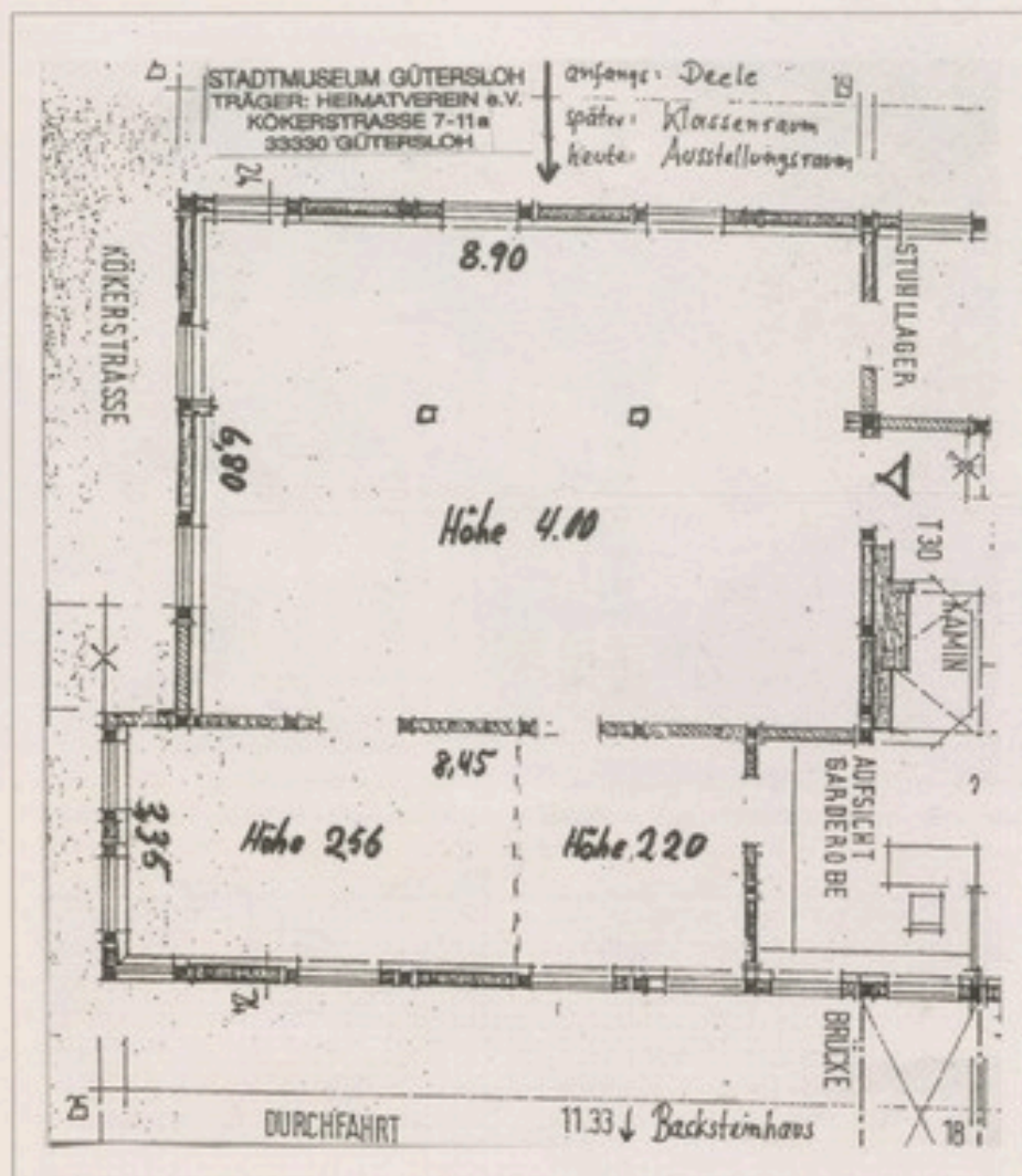
Grundriss dieses Hauses. Foto: Heimatverein Gütersloh
